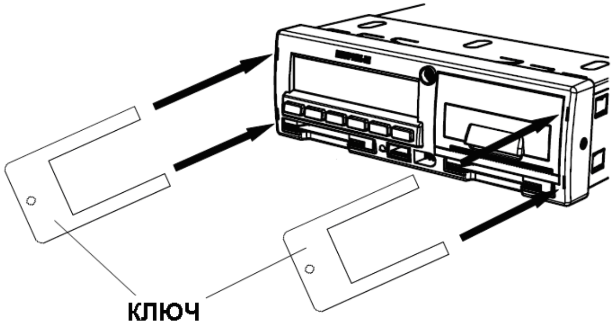
Рисунок 4 – Извлечение тахографа
